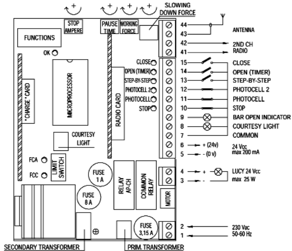
Рисунок 3. Схема разводки
